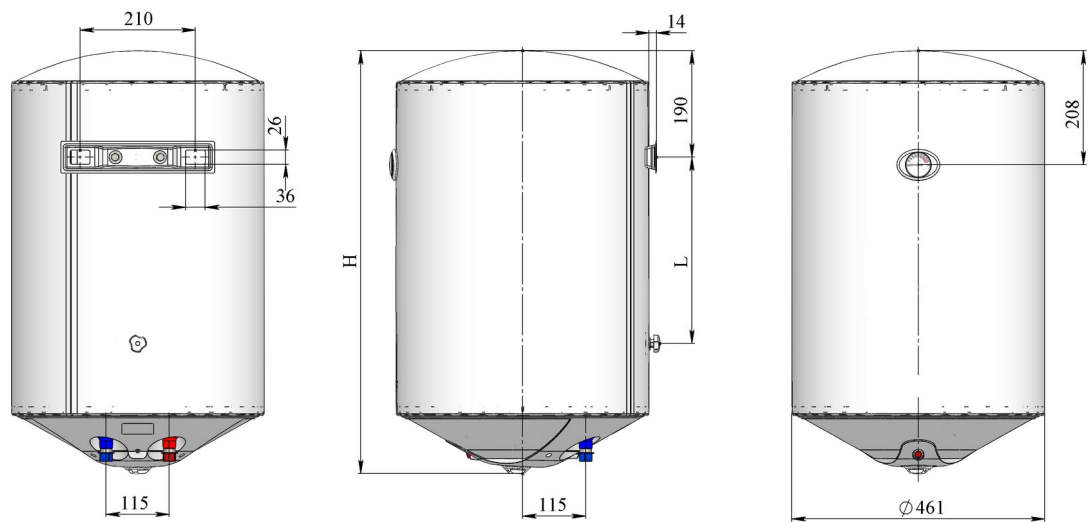
Мал. 2. Монтажні розміри моделей SAM
